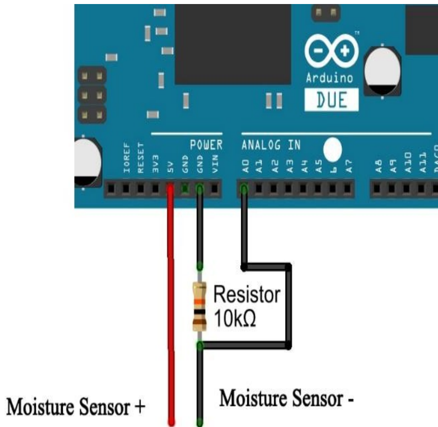
Рисунок 2.13 – Схема підключення датчика вологи
