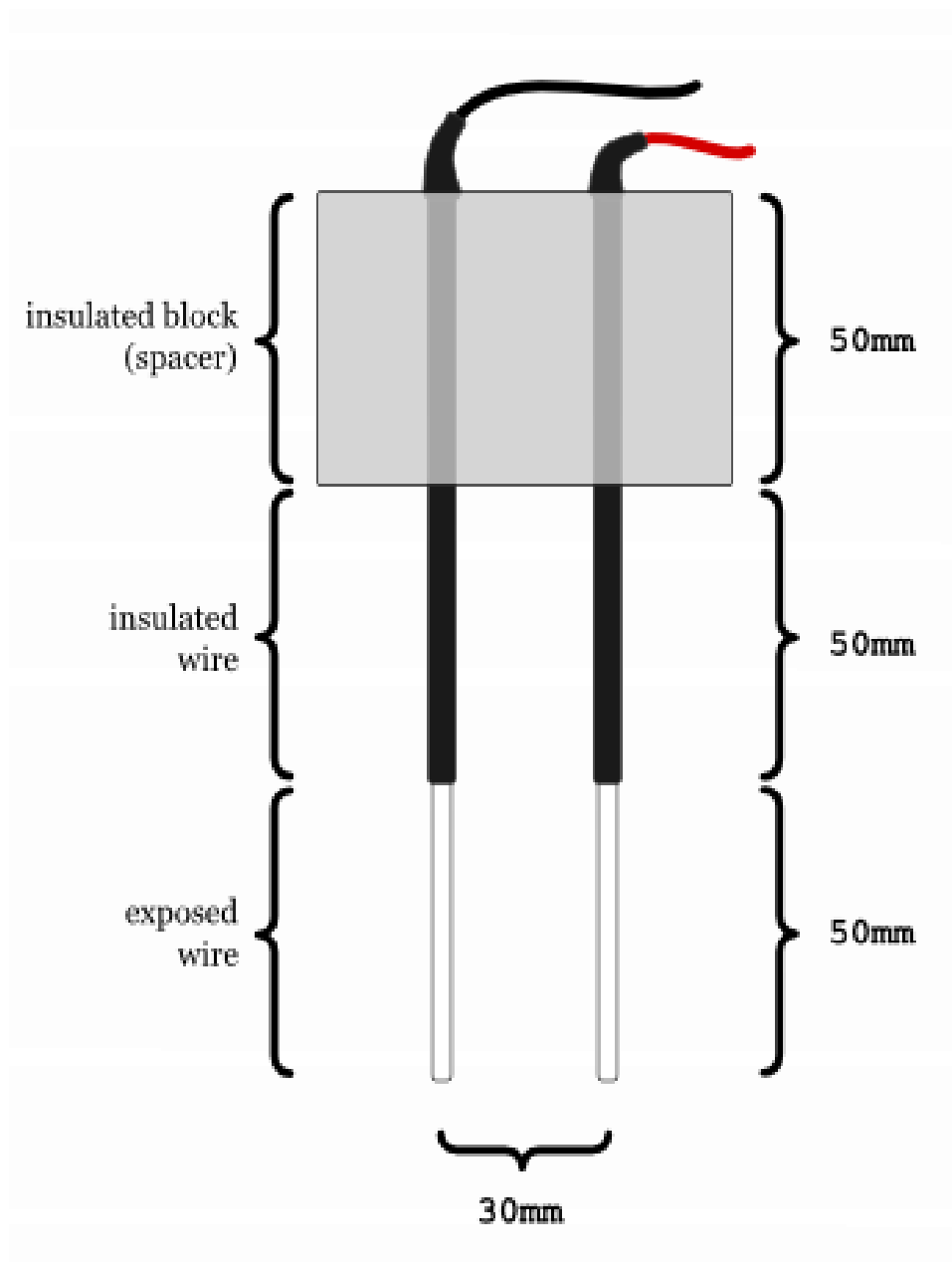
Рисунок 2.12 – Датчик вологості ґрунту
