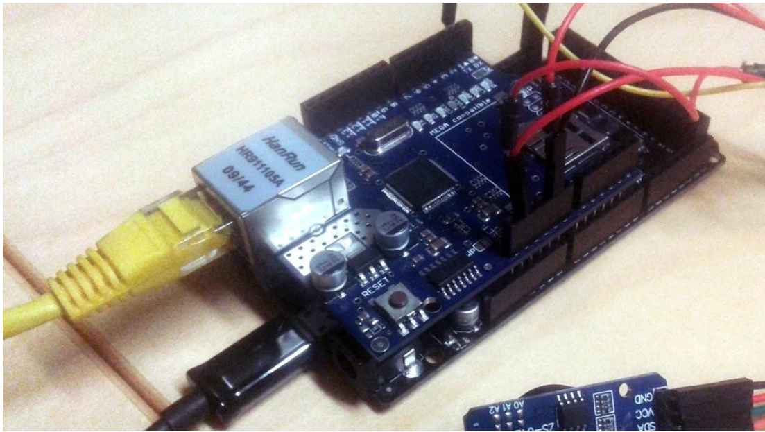
Рисунок 2.3 – Поєднання Ethernet Shield з мікроконтролером Arduino
