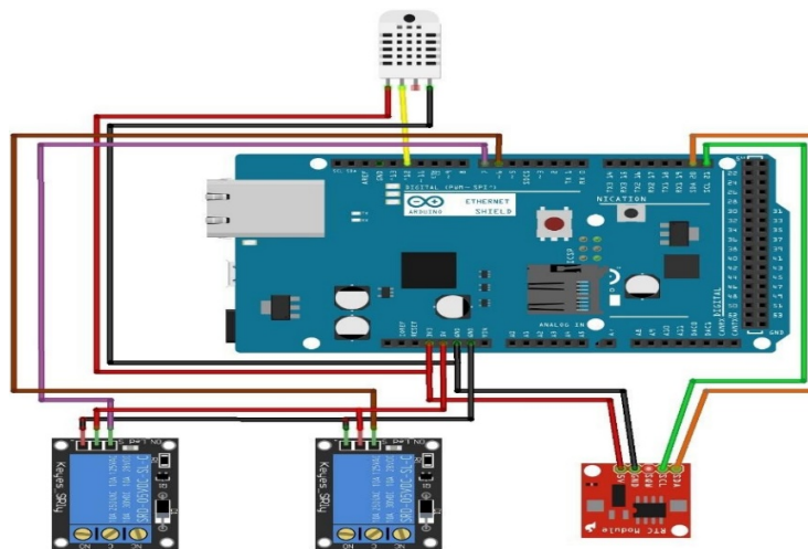
Рисунок 2.14 - Схема підключення обладнання
