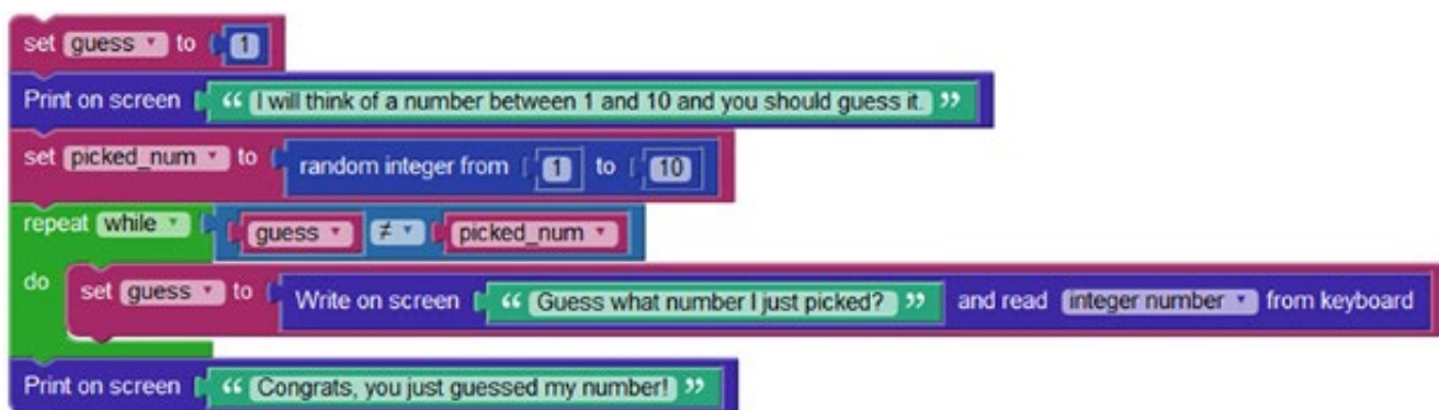
Рисунок 4.5 – Приклада створення гри в Blockly
