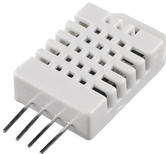
Рисунок 2.4 – Цифровий датчик вологи та температури (DHT22)
