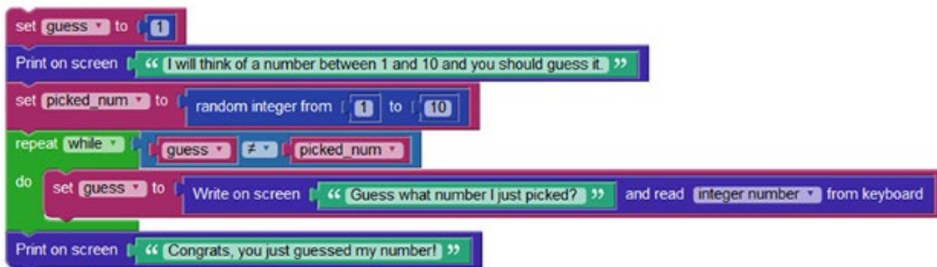
Рисунок 4.6 – Приклад гри вгадування в Blockly
