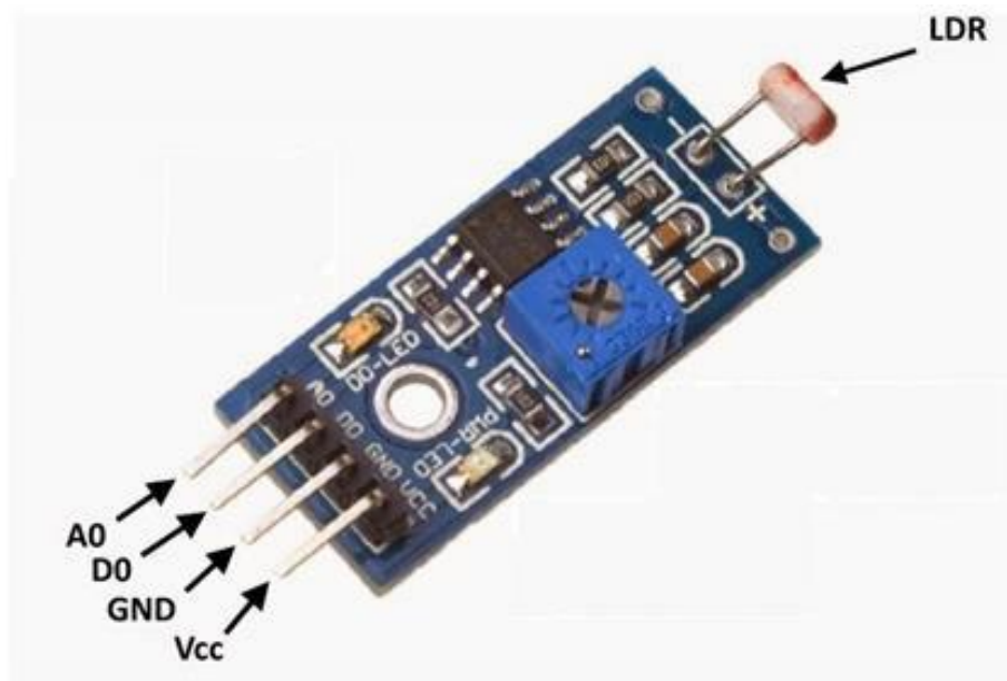
Рисунок 2.7 – Датчик LDR
