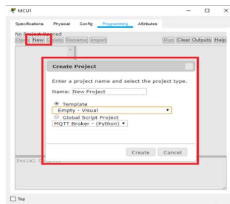
Рис.2. Створення нового проекту в емуляторі Cisco Packet Tracer
