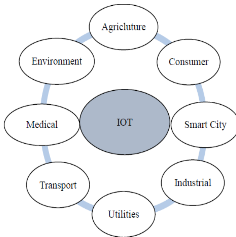
Рисунок 1.4 – Програми IoT
