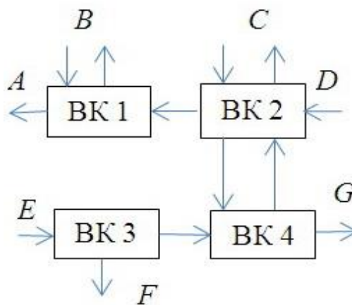
Рис. 1. Приклад мережі
